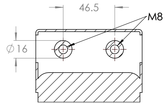
SECTION B-B SCALE 1 : 2
